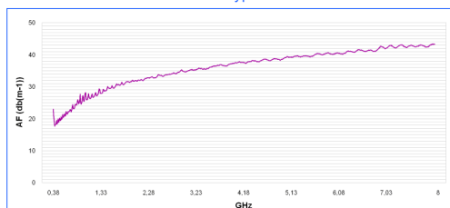
Antennenfaktor HyperLOG 3080
