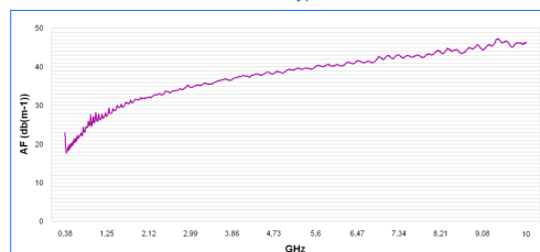
Antennenfaktor HyperLOG 30100
