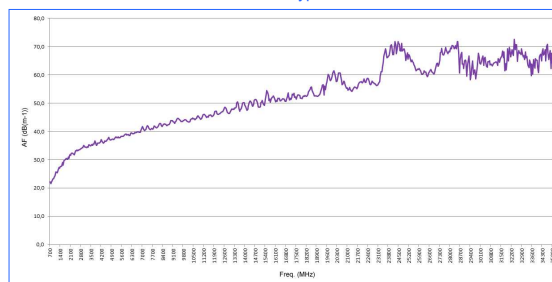
Antennenfaktor HyperLOG 60350
