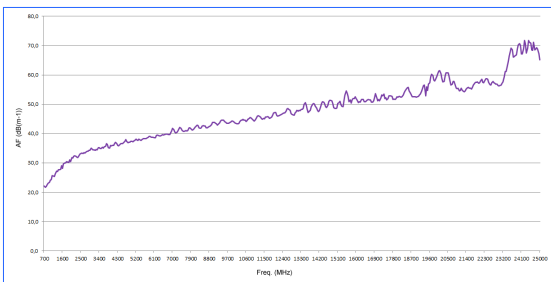
Antennenfaktor HyperLOG 60250
