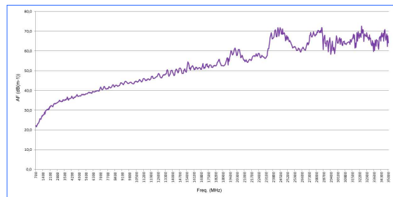
Antennenfaktor HyperLOG 60350
