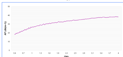
Antennenfaktor HyperLOG 4040
