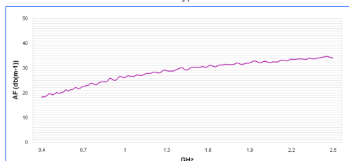
Antennenfaktor HyperLOG 4025
