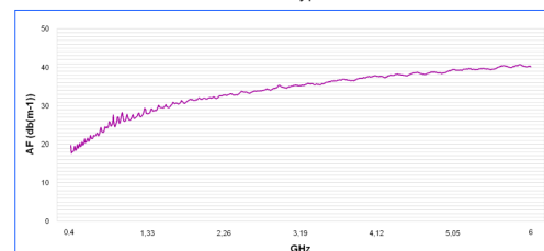
Antennenfaktor HyperLOG 4060
