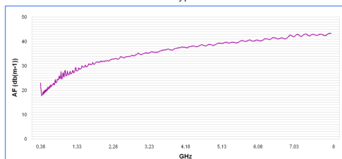
Antennenfaktor HyperLOG 3080
