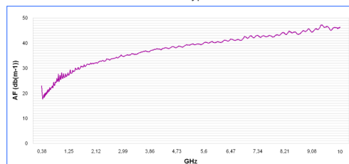
Antennenfaktor HyperLOG 30100
